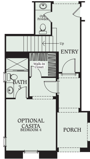
Optional Casita/Powder
